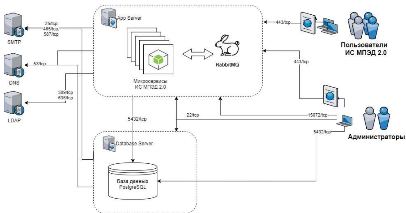
Рисунок 1 Структурная схема ИС МПЭД 2.0
